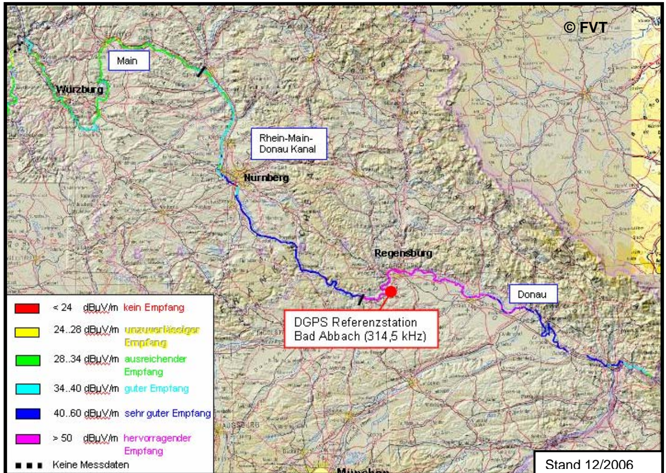
Bild 1: Empfangsfeldstärkewerte der DGPS Referenzstation Bad Abbach
